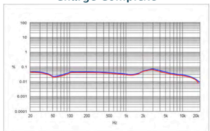
THD + N vs Fréquence: 20W RMS à Charge Complexe
